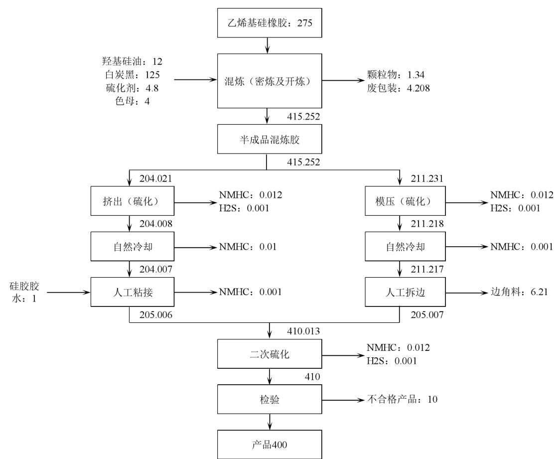
图3.3-1 物料平衡图（t/a）
