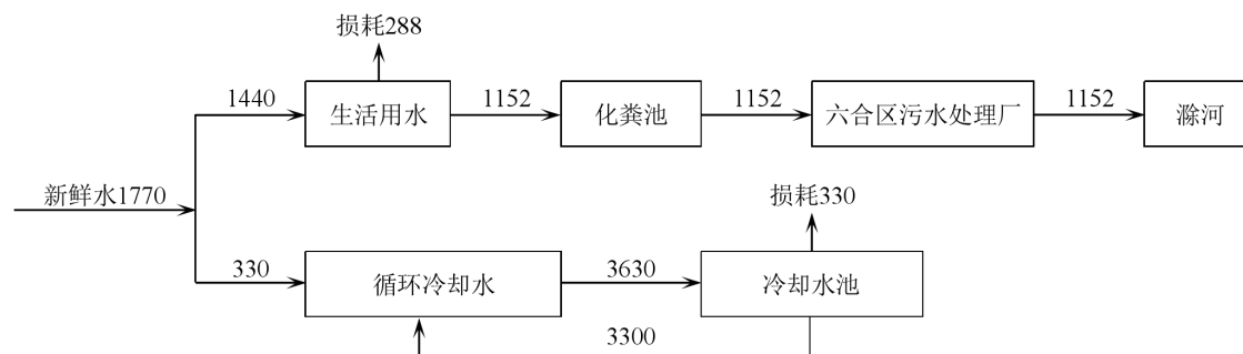
图 3.6-1 水平衡图
