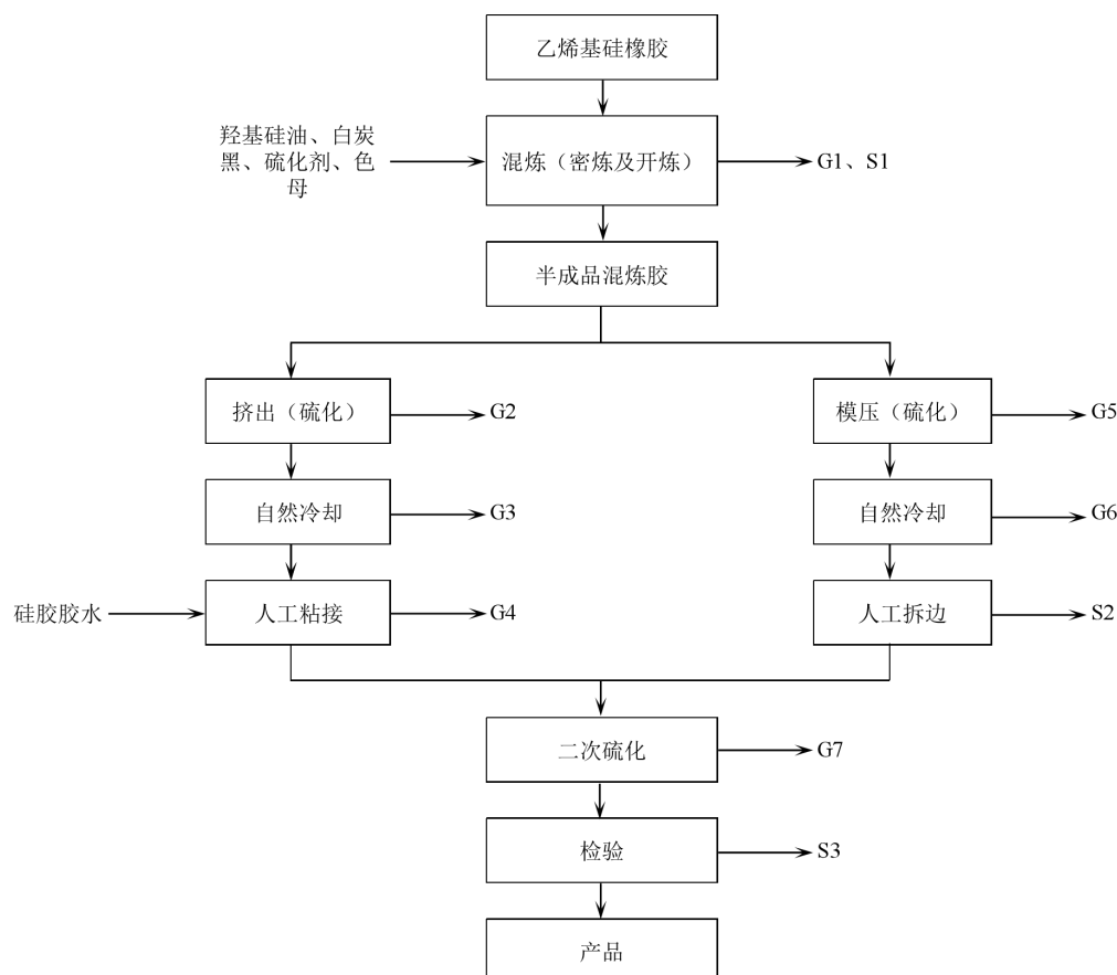
图3.2-1 工艺流程及产物节点图
