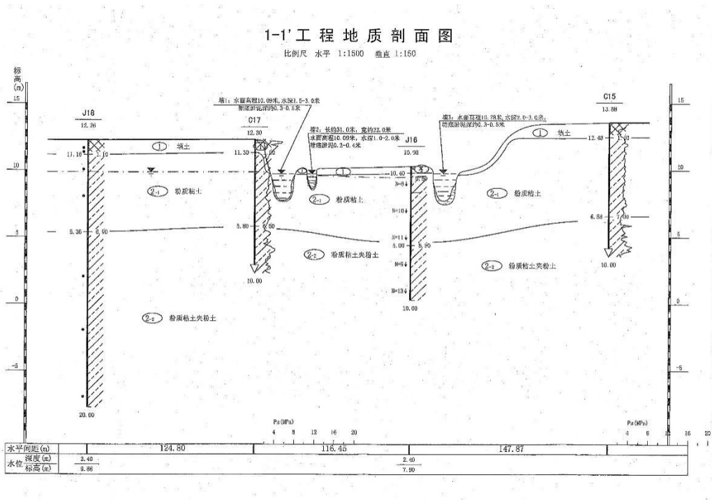
图 5.5-2 区域工程地质剖面图
