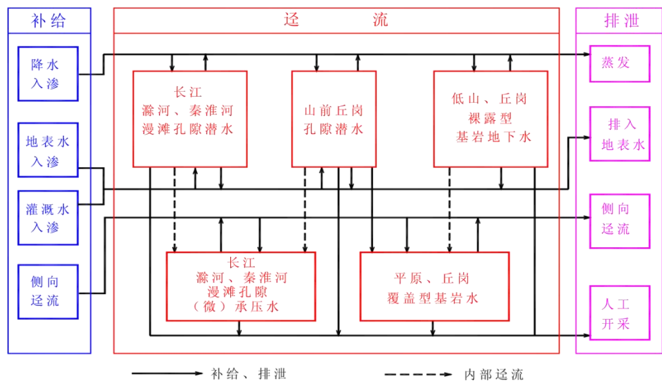
图 5.5-5 地下水补给、径流、排泄关系略图
