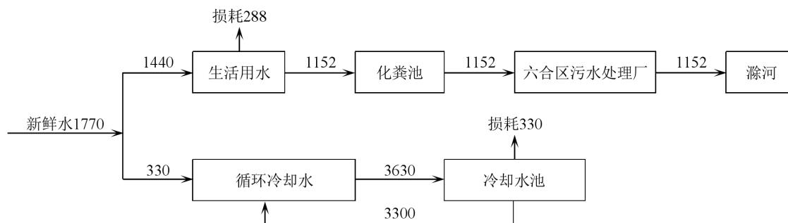
图 3.6-1 水平衡图
