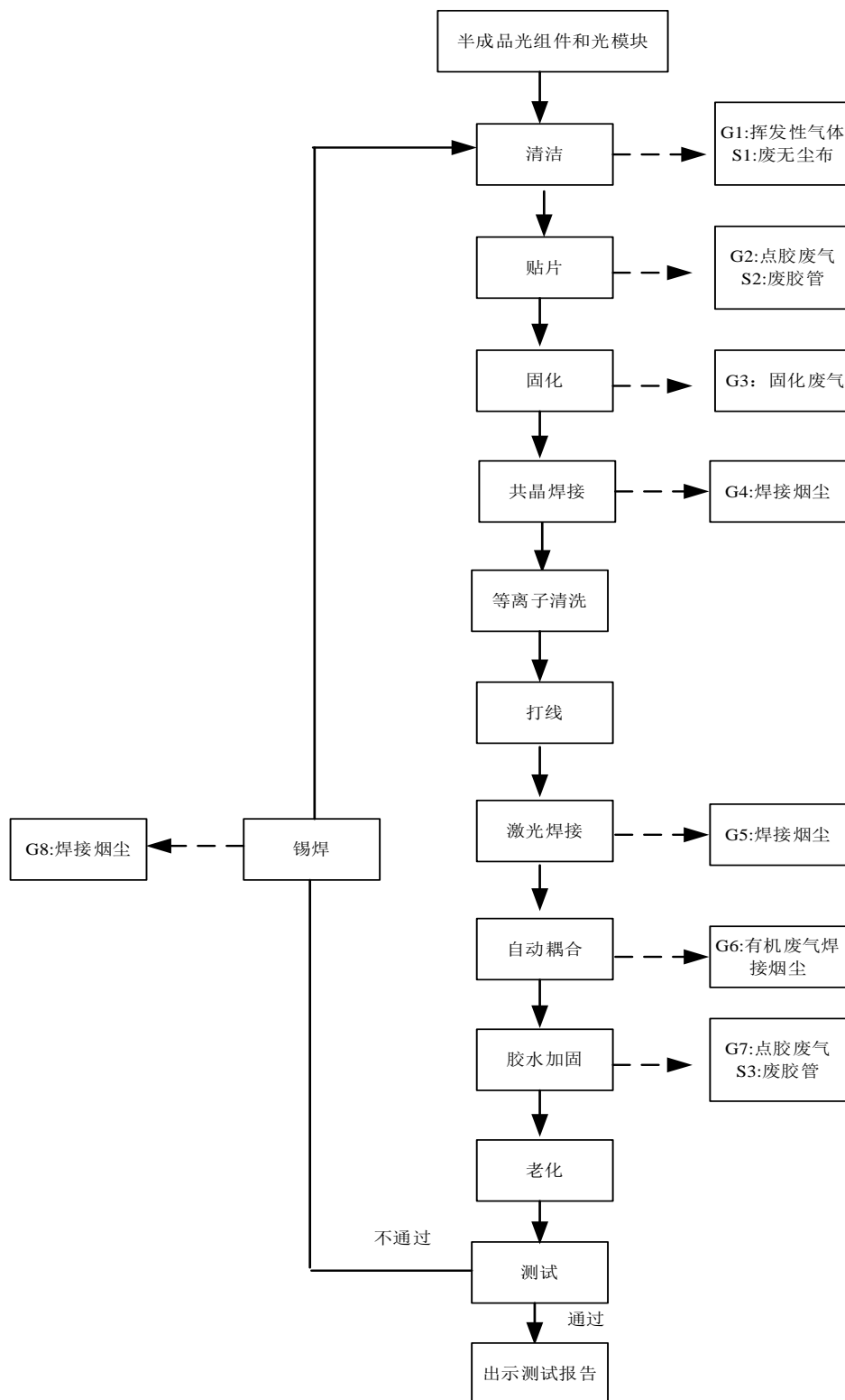
图 5-1 本项目生产工艺流程及产物节点图
