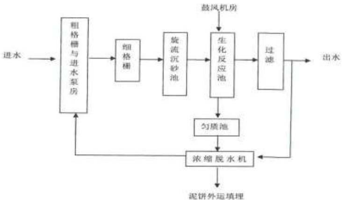
图 7-1 六合区污水处理厂工艺流程图
